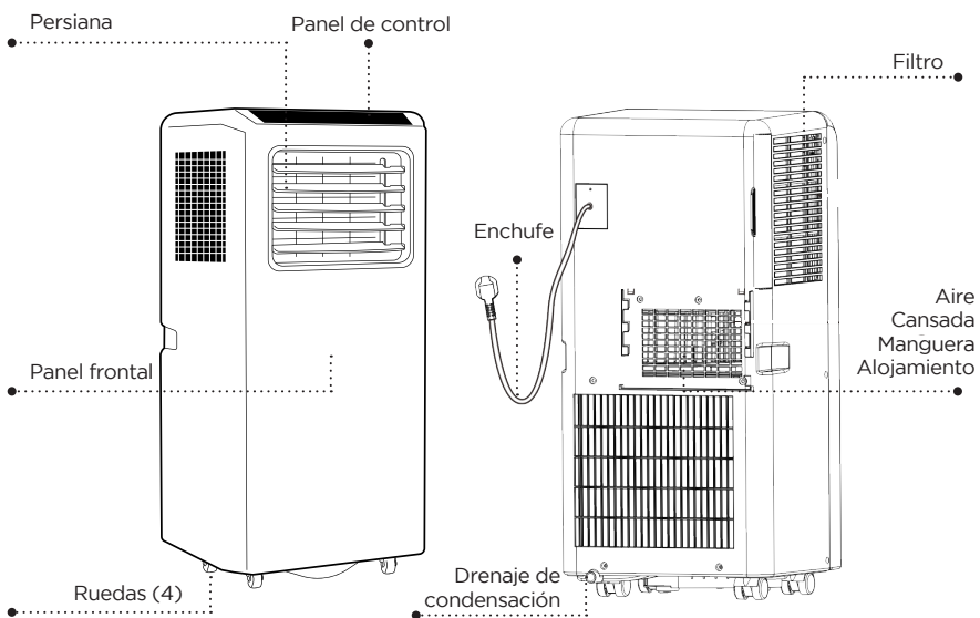
Manquera de evacuación de aire
